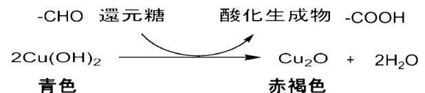
図2. ベネディクト試薬による還元糖の検出
